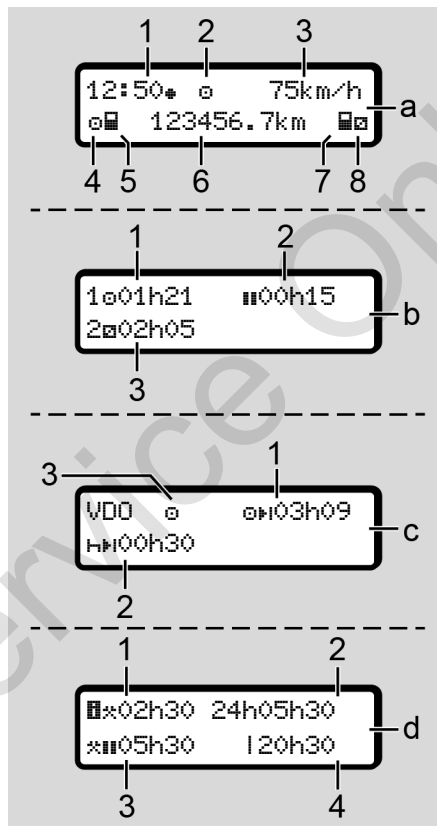
Obr. 8: Standardní obrazovky při jízdě
