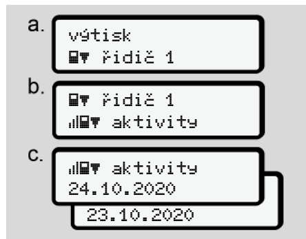
Obr. 88: Posloupnost výtisku – aktivity
