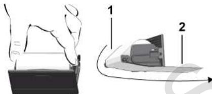
Obr. 126: Vložení role papíru
