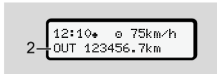
Obr. 118: Standardní zobrazení - Out of scope
