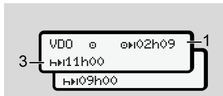
Obr. 64: Aktivita 0 – zbyvájící doba řízení vs. denní doba odpočinku
