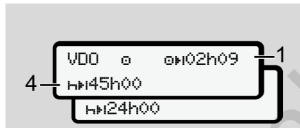
Obr. 65: Aktivita 0 – zbyvájící doba řízení vs. týdenní doba odpočinku
