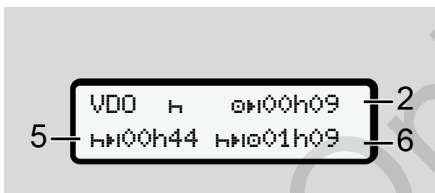
Obr. 69: Aktivita H – doba odpočinku vs. použitelná denní doba řízení
