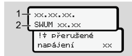
Obr. 130: Zobrazení - přerušení napětí
