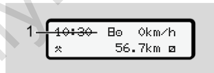
Obr. 117: Standardní zobrazení – stav výroby
