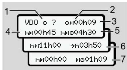
Obr. 62: VDO Counter – uspořádání displeje
